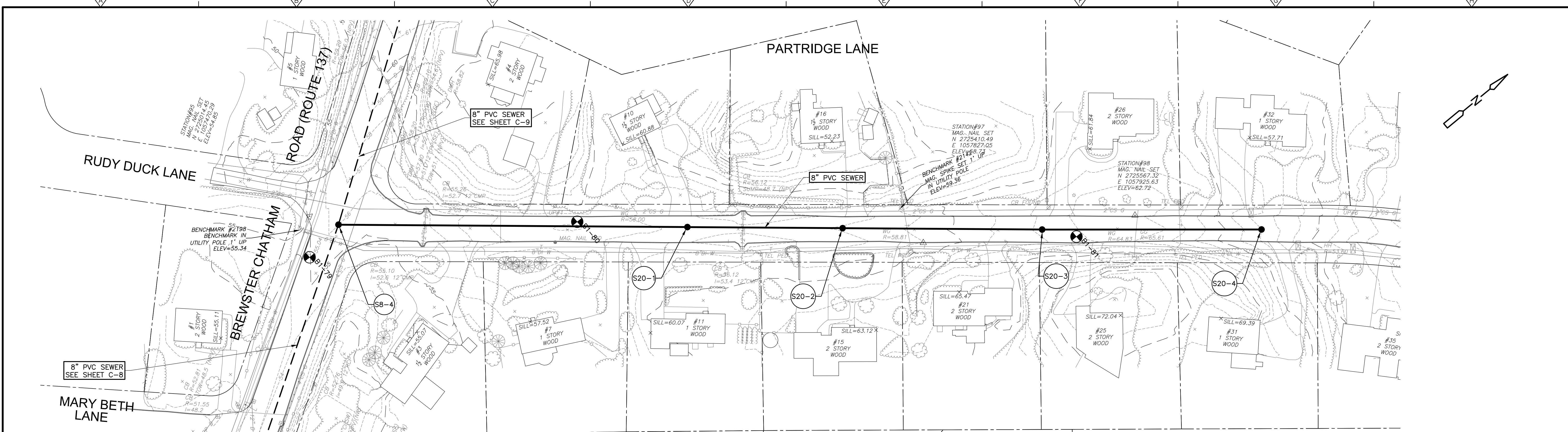
PLAN SCALE: 1"=40'-0"
