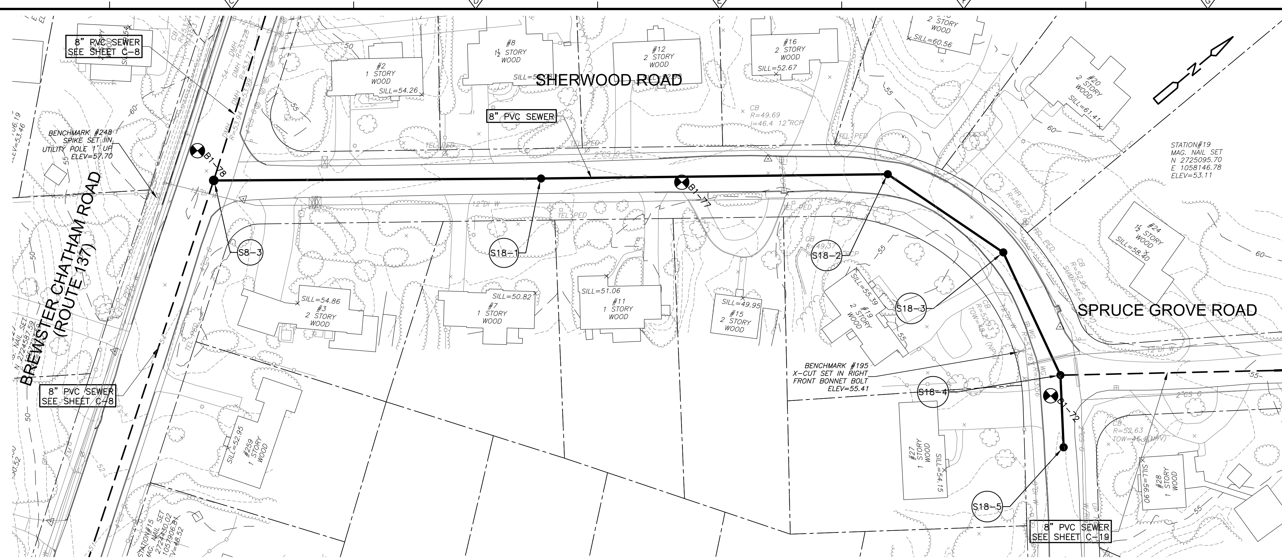
PLAN SCALE: 1"=40'-0"
