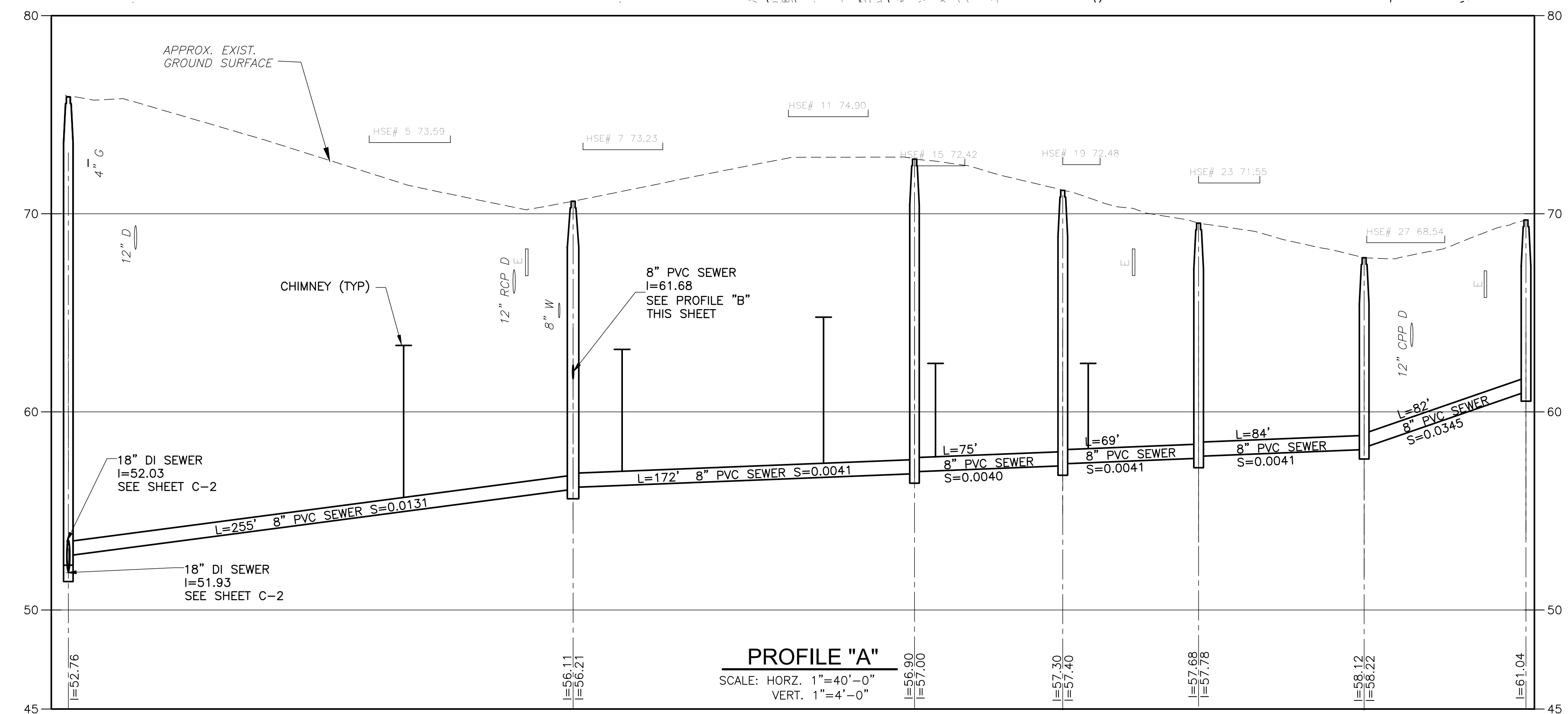
PLAN SCALE: 1"=40'-0"
