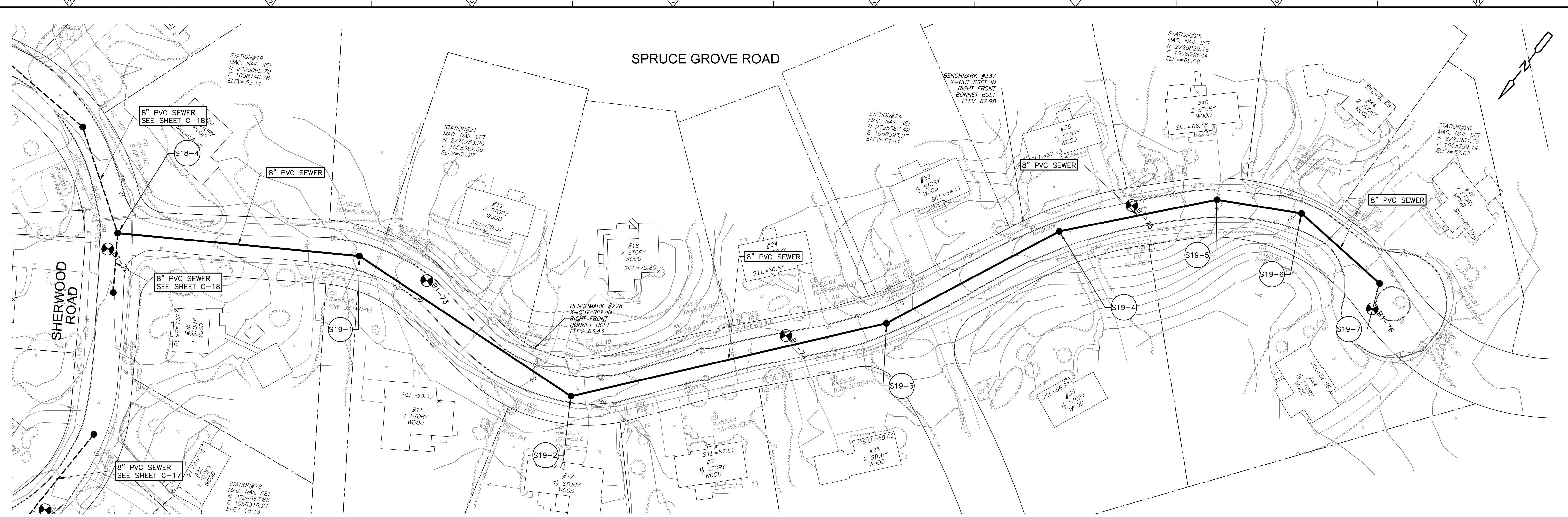
PLAN SCALE: 1"=40'-0"
