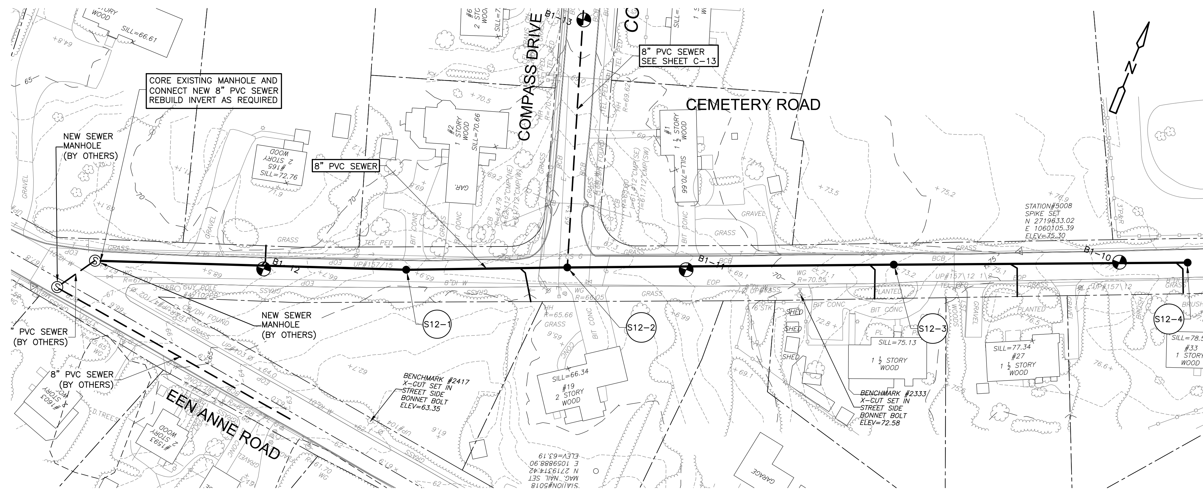
PLAN SCALE: 1"=40'-0"
