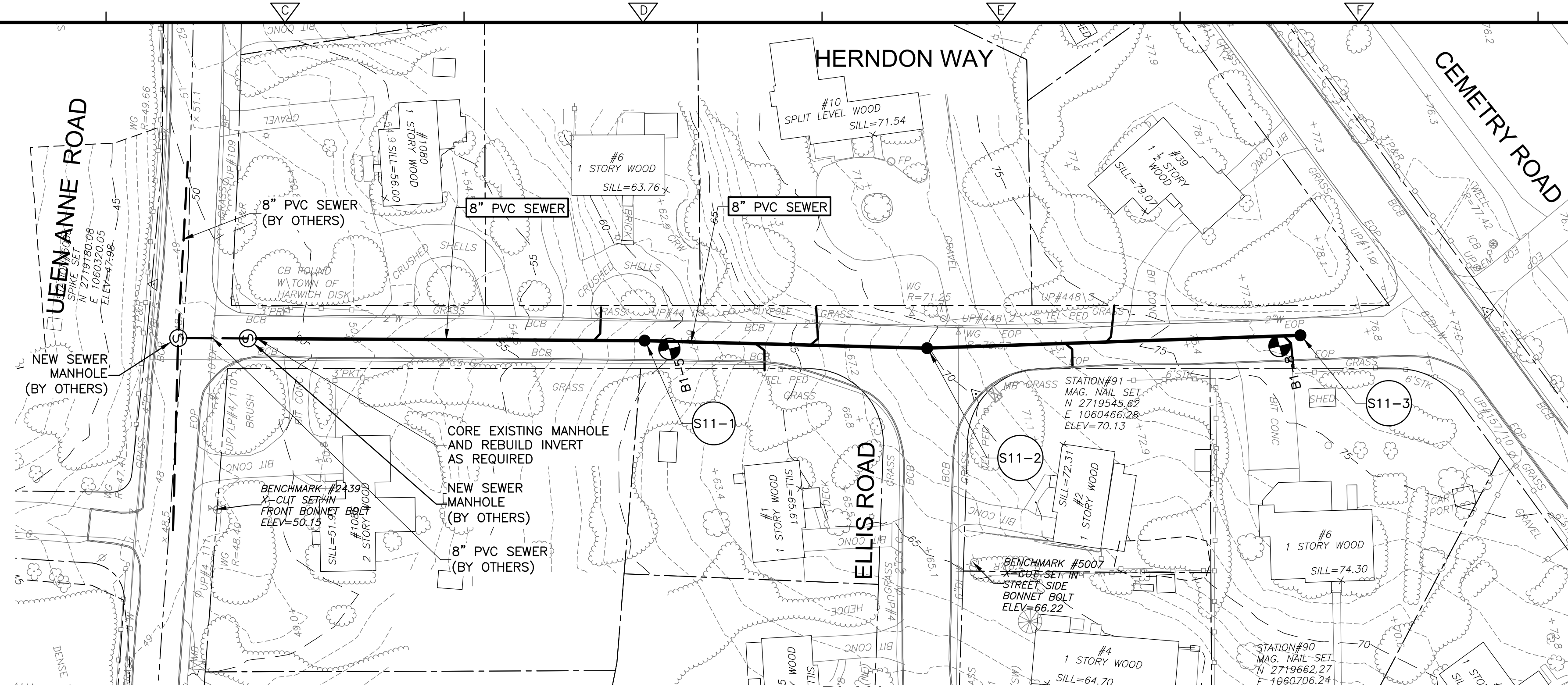
PLAN SCALE: 1"=40'-0"
